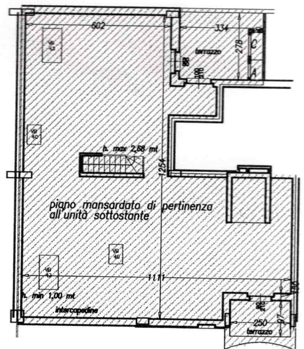
PIANTA PIANO MANSARDA destinazione: RESIDENZA D3s
