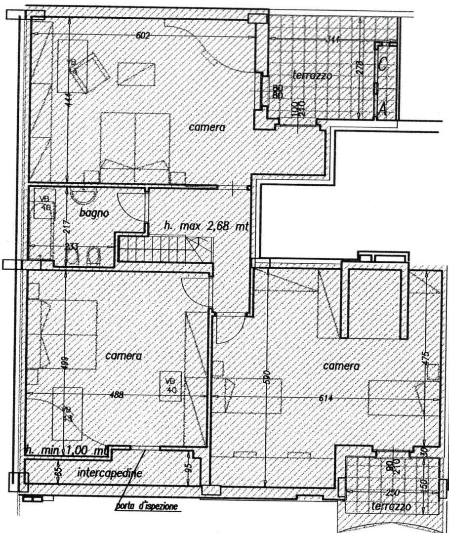
D3s PIANTA PIANO MANSARDA destinazione: RESIDENZA DISPOSIZIONE PROPOSTA
